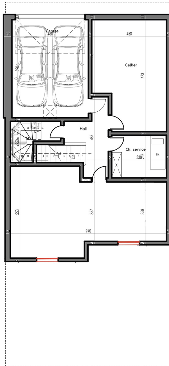
PLAN SOUS SOL
