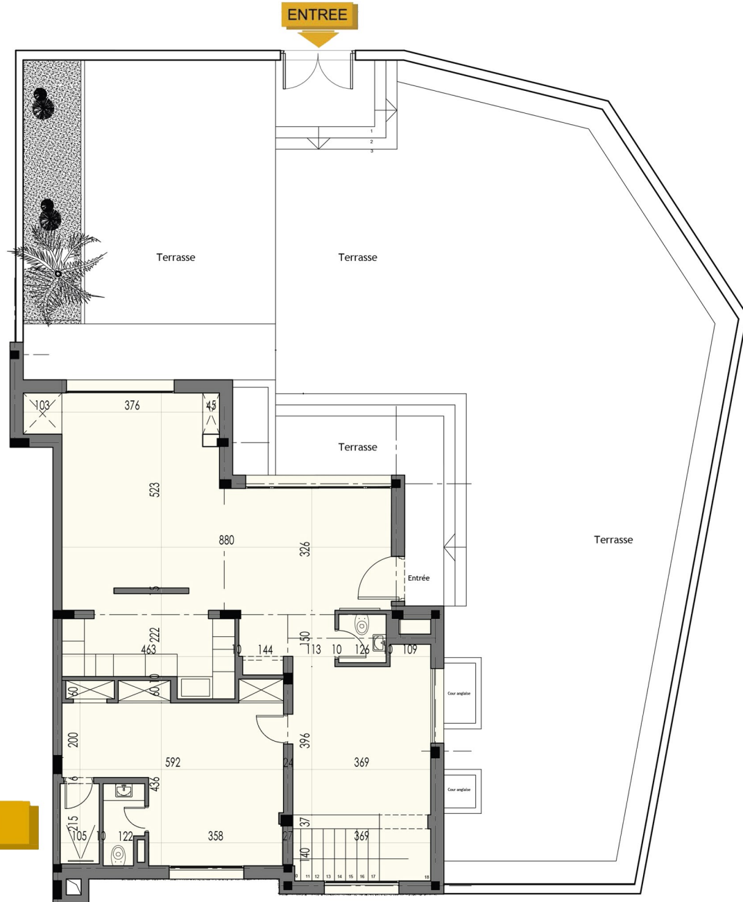
PLAN REZ DE CHAUSSEE
